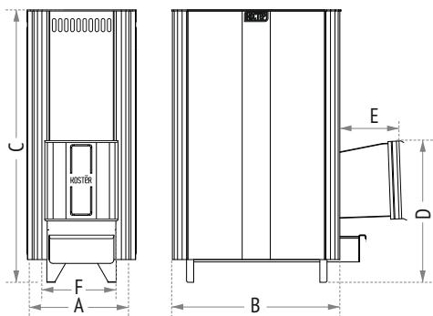
Печи с выносным топливным каналом
